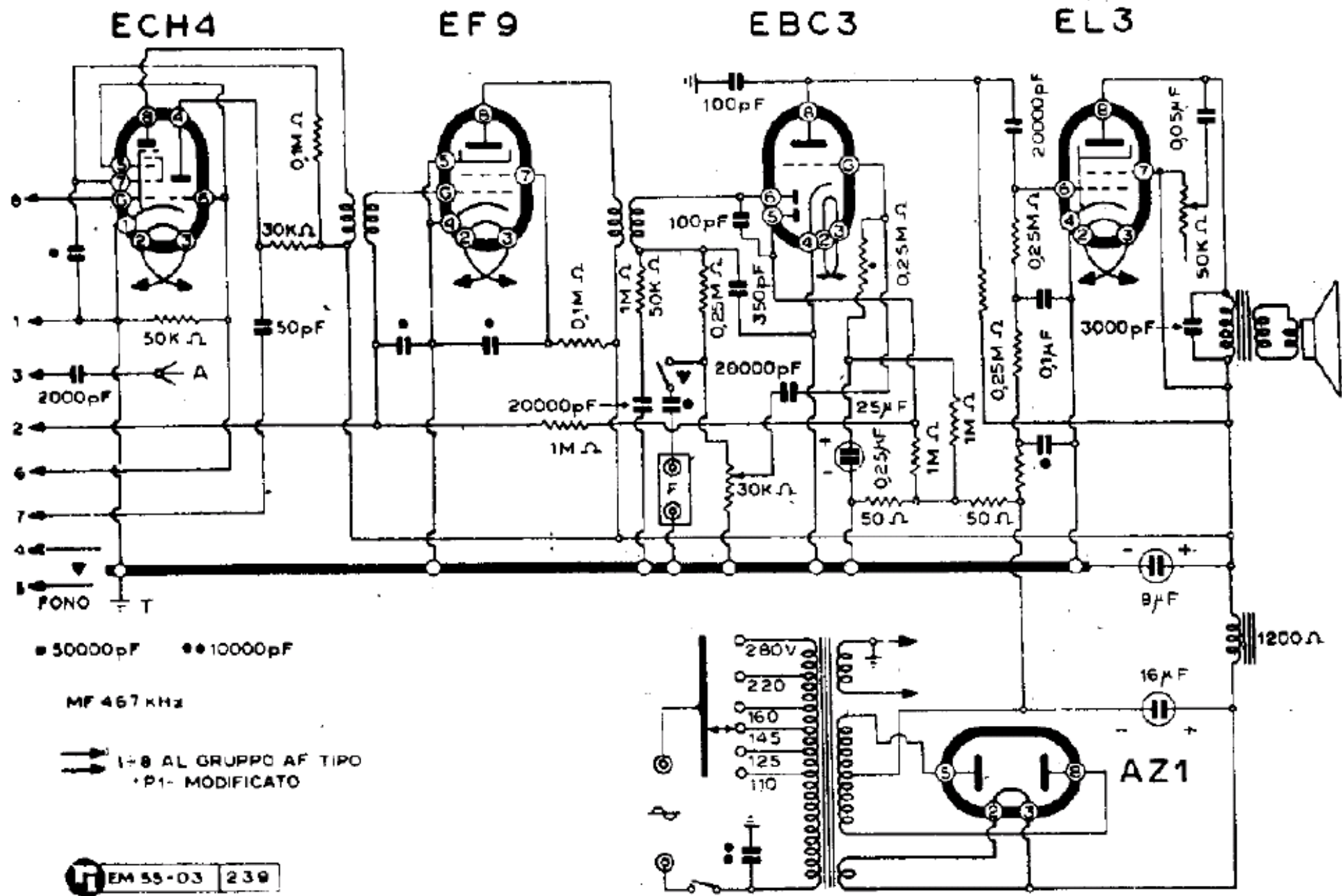
ELECTA RADIO - MOD. « ER 556-L »
